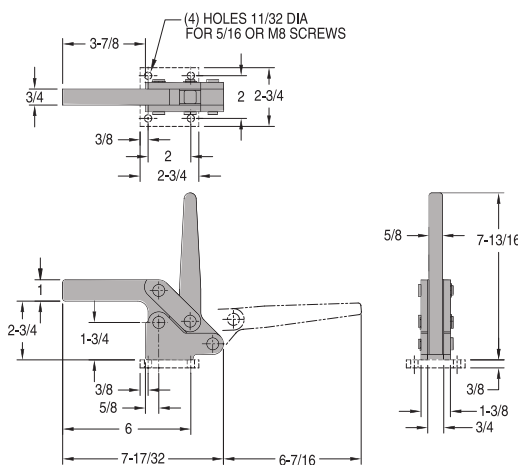
CL-61-HDC-211
