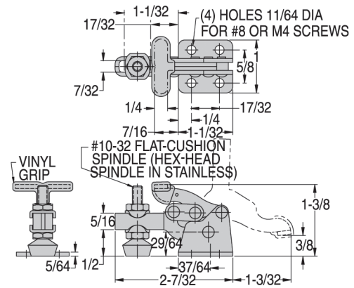
CL-200-VTC
