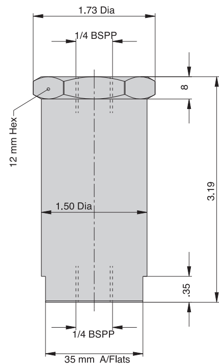
CLR-3887-087
