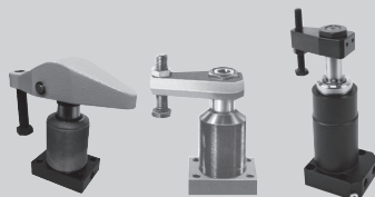
Flange Base pages 615-616
