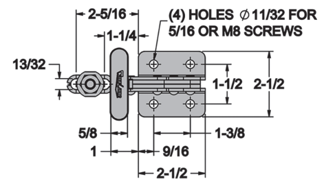
CL-300-VTC
