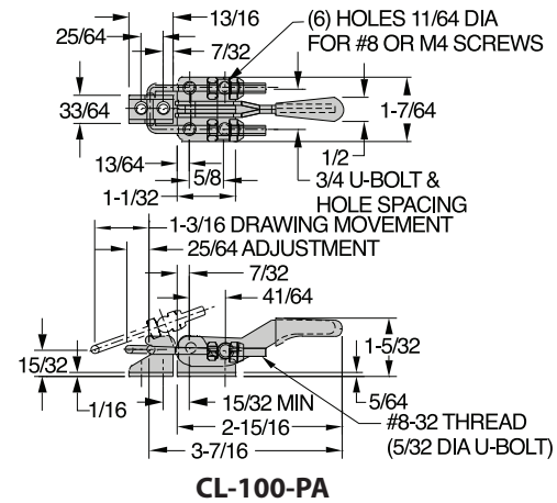
CL-100-PA
