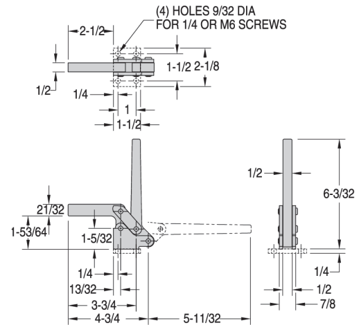
CL-40-HDC-211
