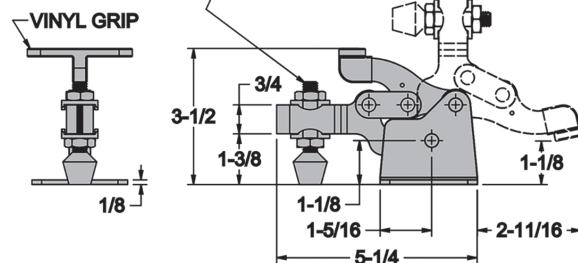
CL-500-VTC
