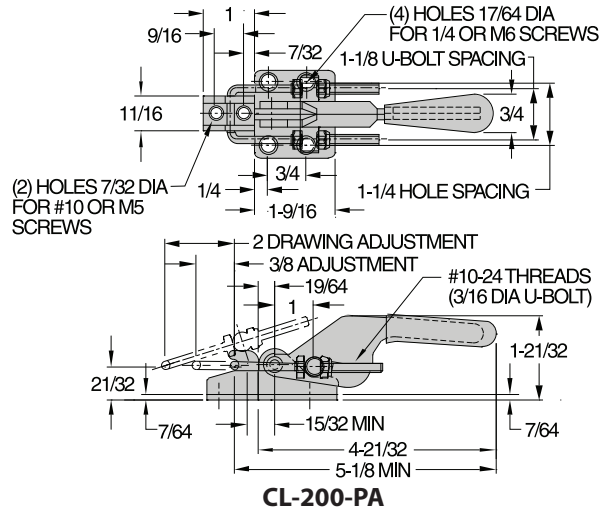
CL-200-PA
